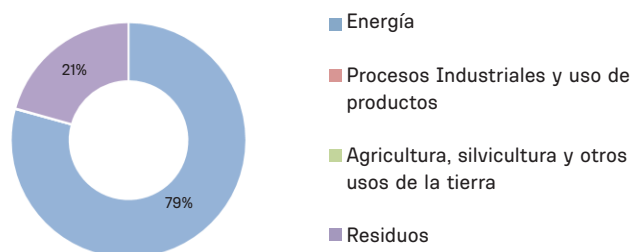
Figura 4: Emisiones totales CO 2 eq por sector (en porcentaje), 2021.
