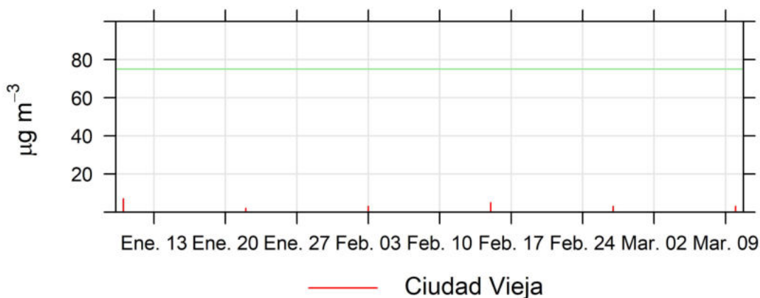
Ilustración 2.1 - Resultados de Humo Negro de la estación Ciudad Vieja
