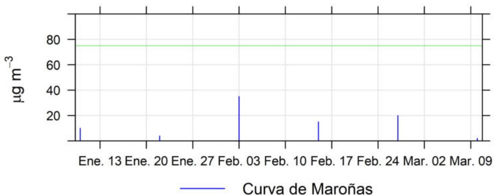
Ilustración 2.9- Resultados HN de la estación Curva de Maroñas
