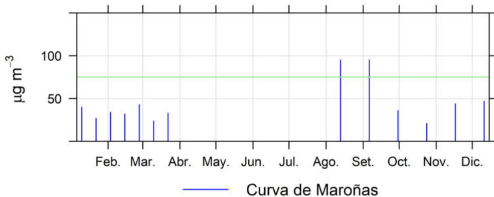
Ilustración 2.8 - Resultados PM10 (manual) de la estación Curva de Maroñas
