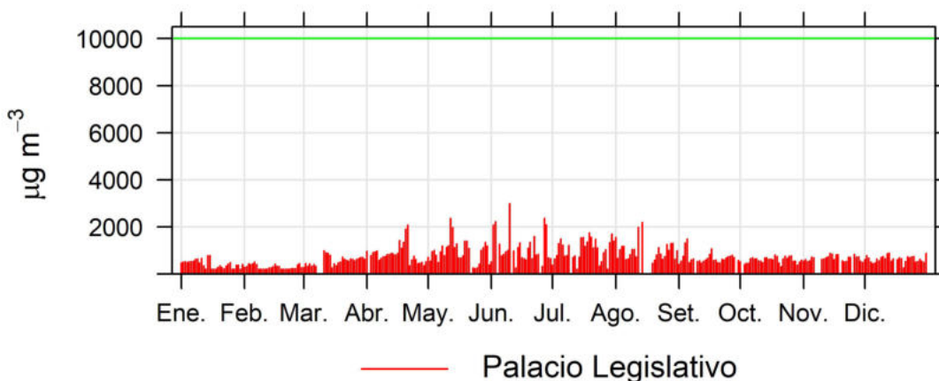
Ilustración 2.20 - Resultados CO de la estación Palacio Legislativo
