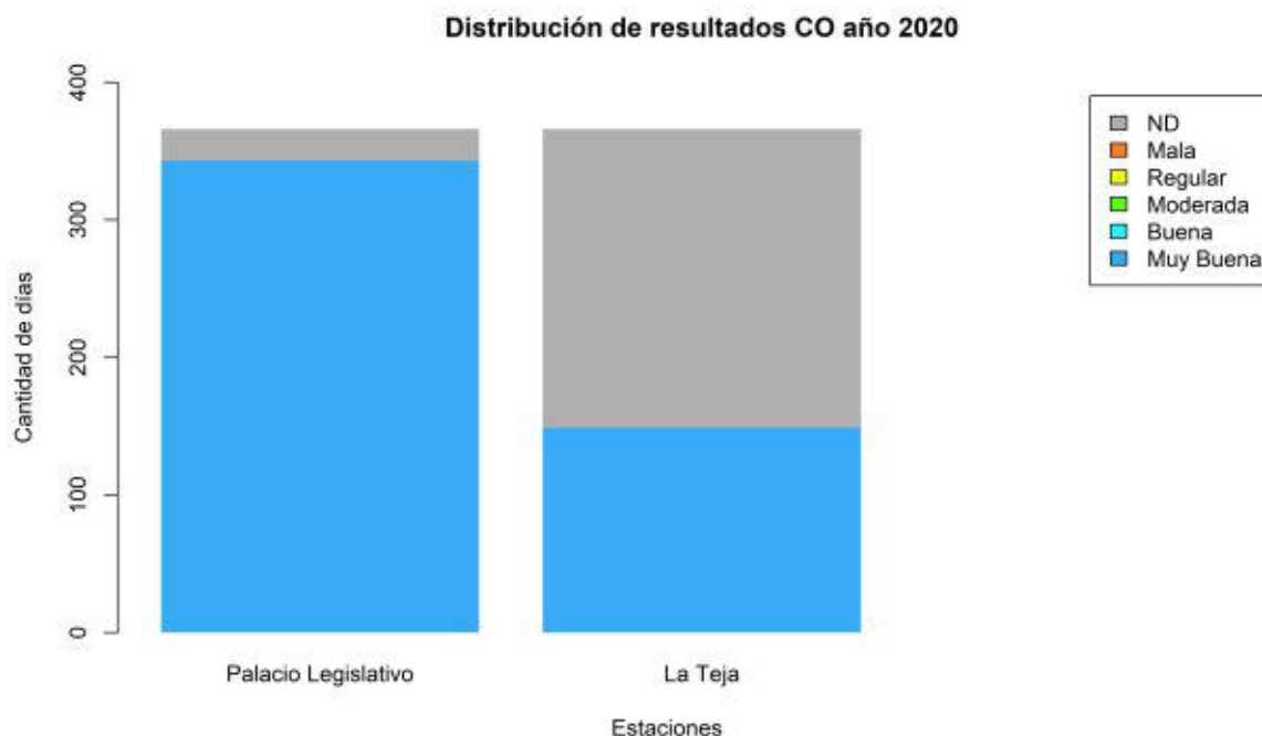
Ilustración 3.16 - Distribución por categorías CO 2020 por estación
