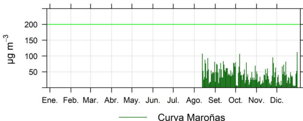
Ilustración 2.6 - Resultados NO 2 de la estación Curva de Maroñas
