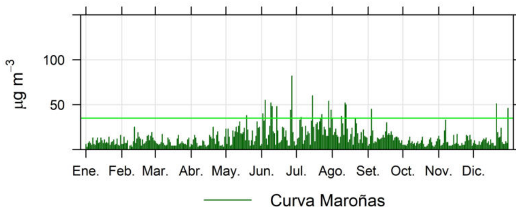
Ilustración 2.5 - Resultados PM 2.5 de la estación Curva de Maroñas
