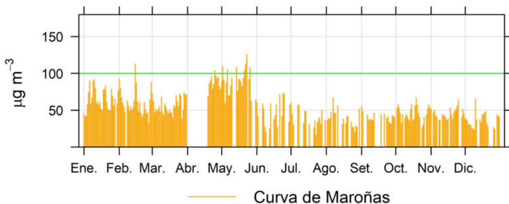
Ilustración 2.7 - Resultados O 3 de la estación Curva de Maroñas
