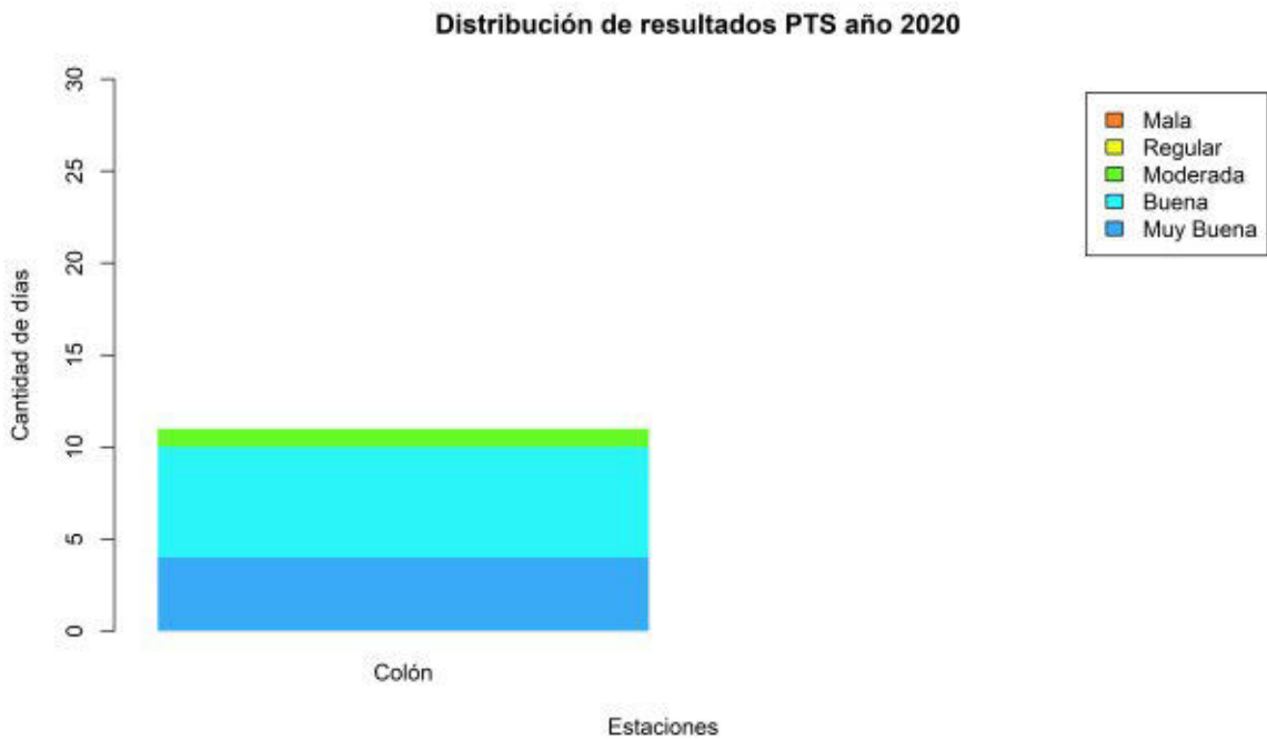
Ilustración 3.2 - Distribución por categorías PTS 2020 por estación
