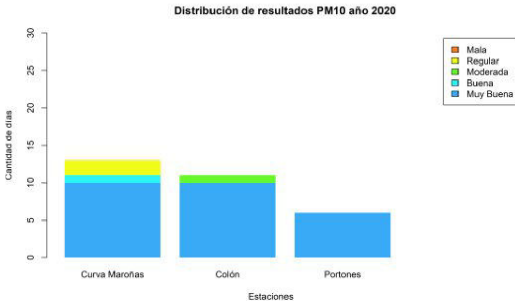
Ilustración 3.4 - Distribución por categorías PM10 manual 2020 por estación
