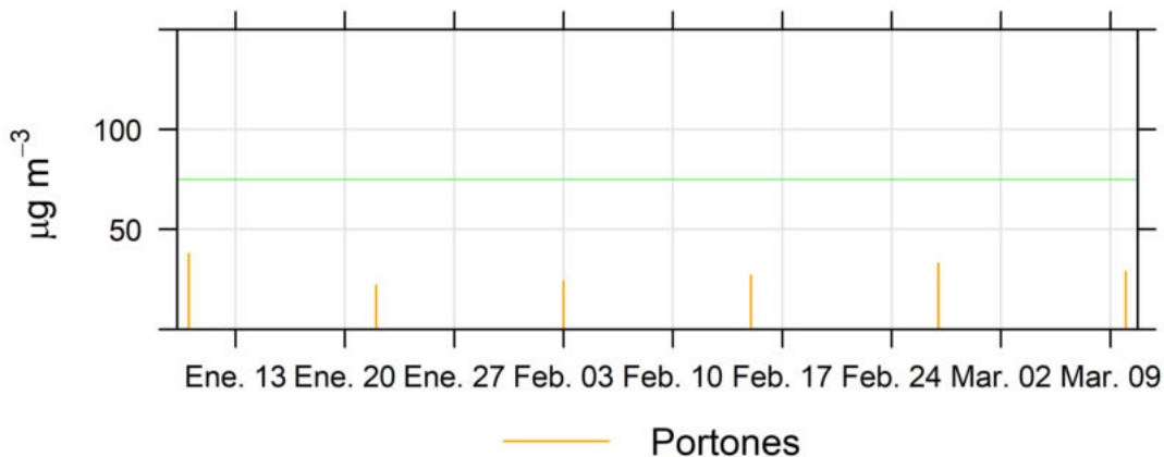
Ilustración 2.10 - Resultados PM10 (manual) de la estación Portones de Carrasco
