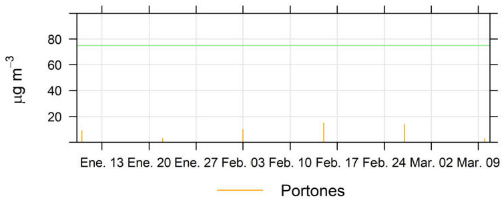
Ilustración 2.11 - Resultados HN de la estación Portones de Carrasco
