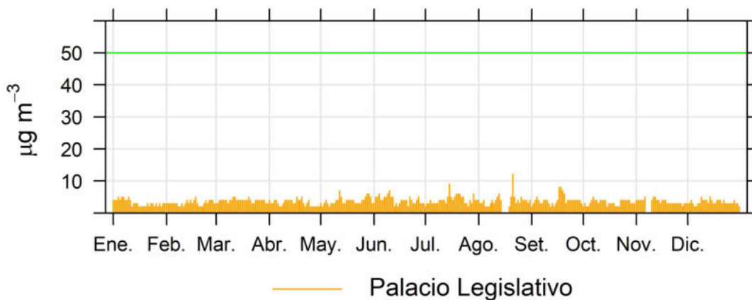
Ilustración 2.19 - Resultados SO 2 de la estación Palacio Legislativo
