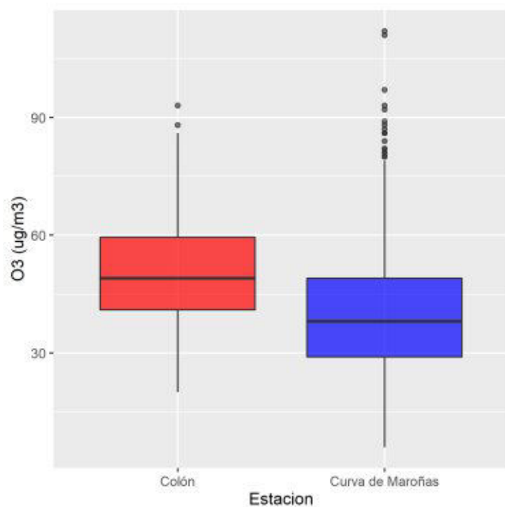
Ilustración 3.19 - Gráfico de cajas O3 2020 por estación
