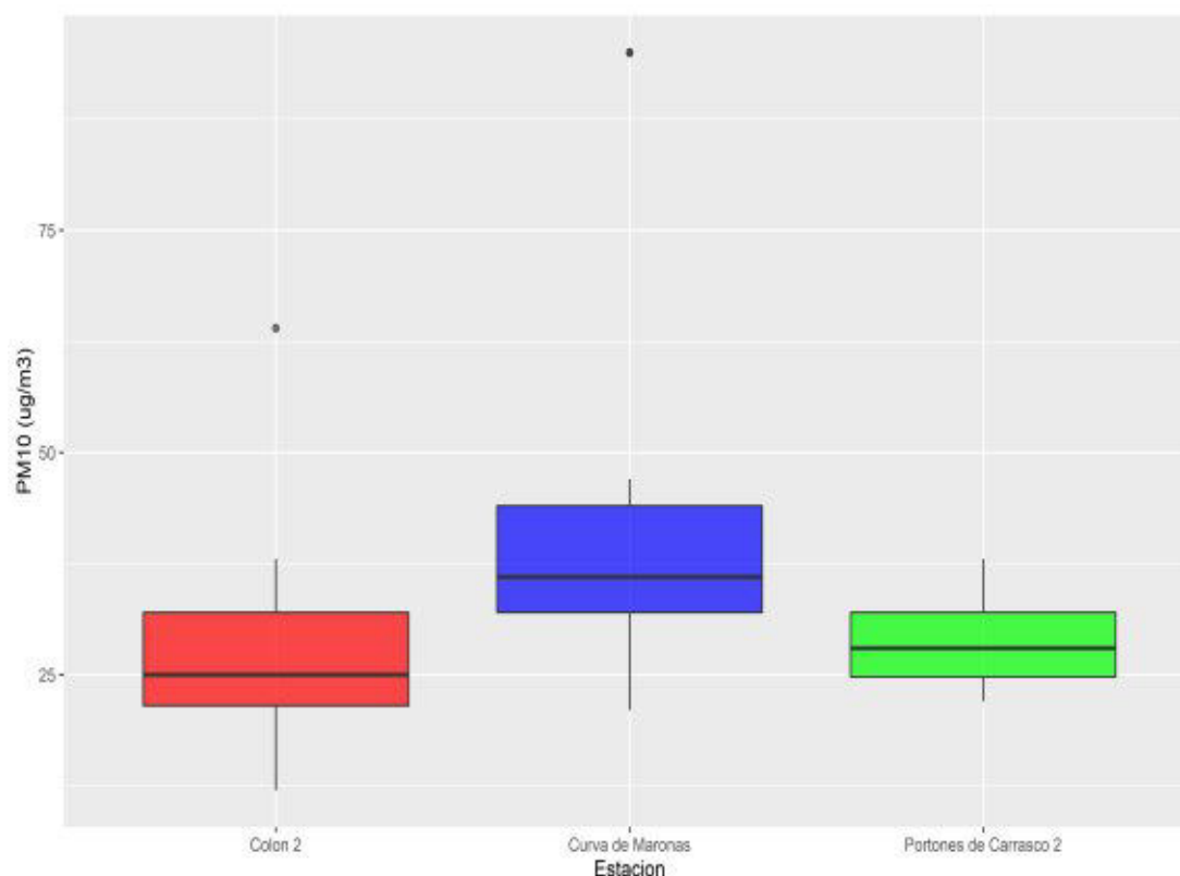
Ilustración 3.3 - Gráfico de cajas PM10 manuales 2020 por estación
