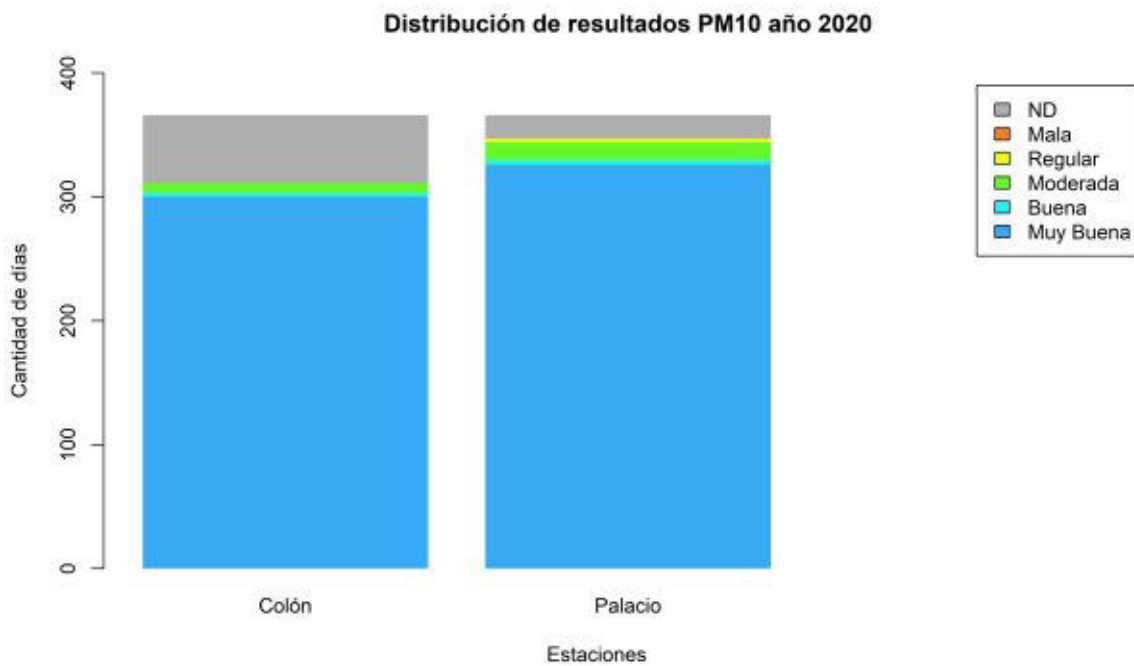
Ilustración 3.6 - Distribución por categorías PM10 2020 por estación
