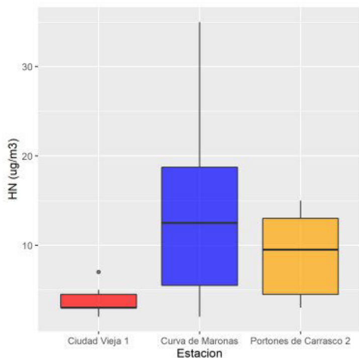
Ilustración 3.9 - Gráfico de cajas HN 2020 por estación
