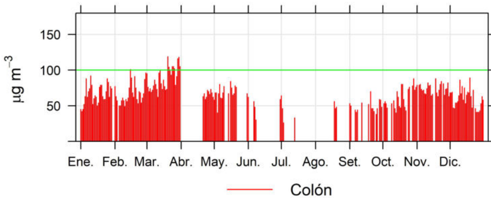
Ilustración 2.13 - Resultados O3 de la estación Colón
