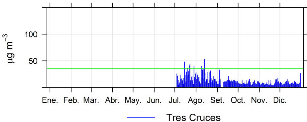
Ilustración 2.3 - Resultados PM 2.5 de la estación Tres Cruces
