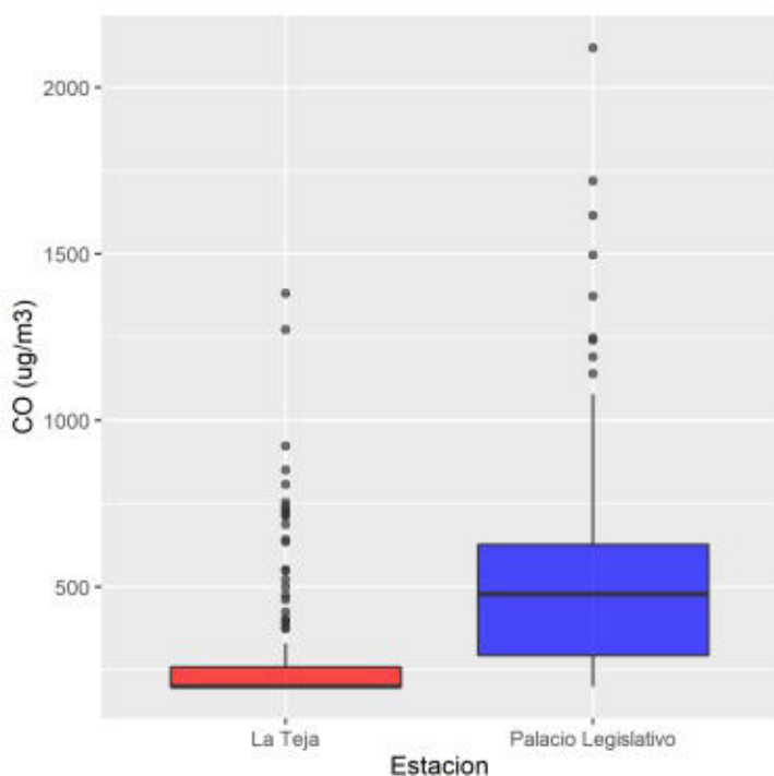
Ilustración 3.15 - Gráfico de cajas CO 2020 por estación
