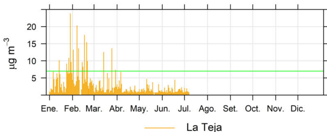
Ilustración 2.24 - Resultados TRS de la estación La Teja
