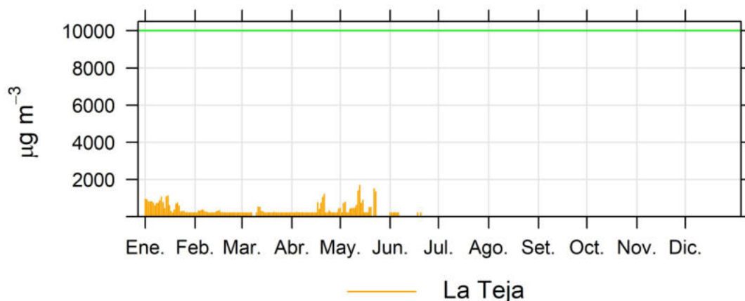
Ilustración 2.22 - Resultados CO de la estación La Teja
