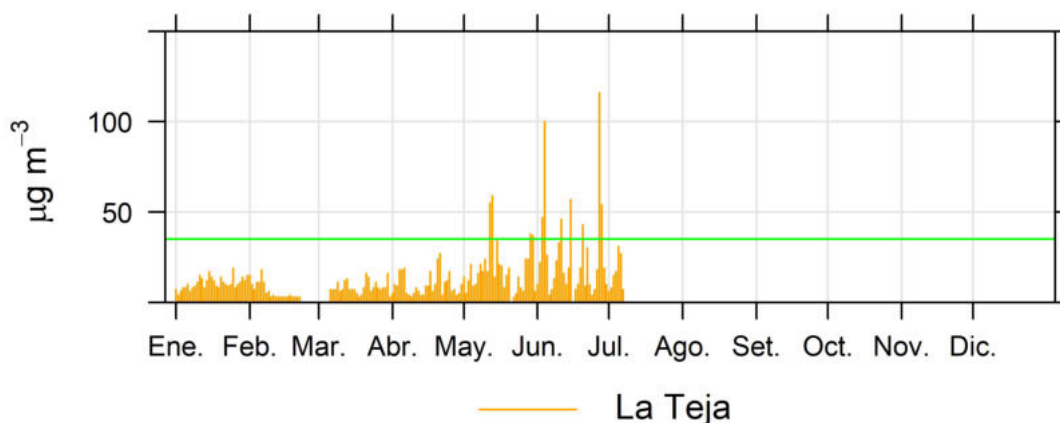
Ilustración 2.21 - Resultados PM2.5 de la estación La Teja
