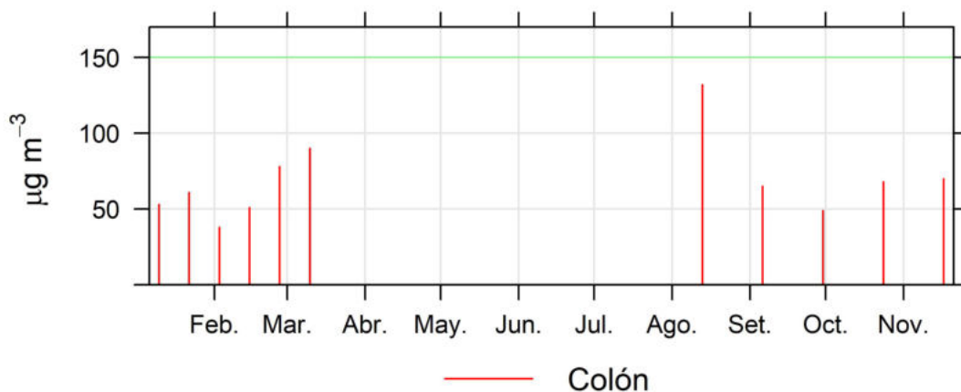
Ilustración 2.16- Resultados PTS (manual) de la estación Colón
