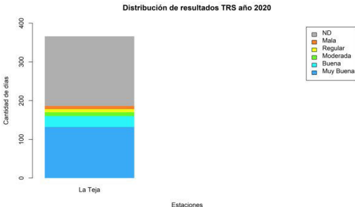
Ilustración 3.18 - Distribución por categorías TRS 2020 por estación
