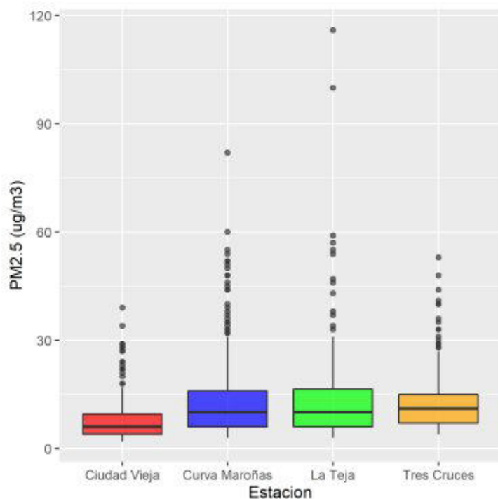
Ilustración 3.7 - Gráfico de cajas PM2.5 2020 por estación
