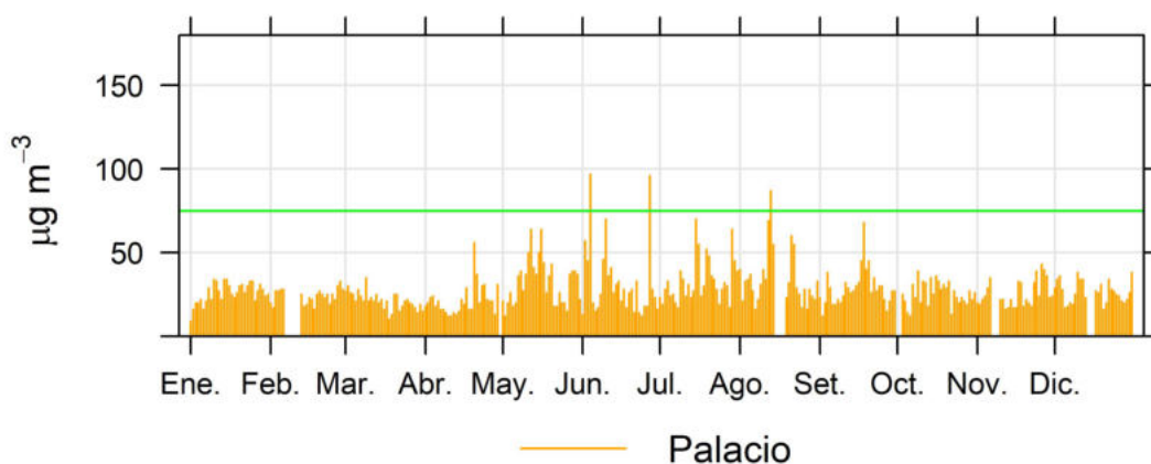
Ilustración 2.17 - Resultados PM10 de la estación Palacio Legislativo
