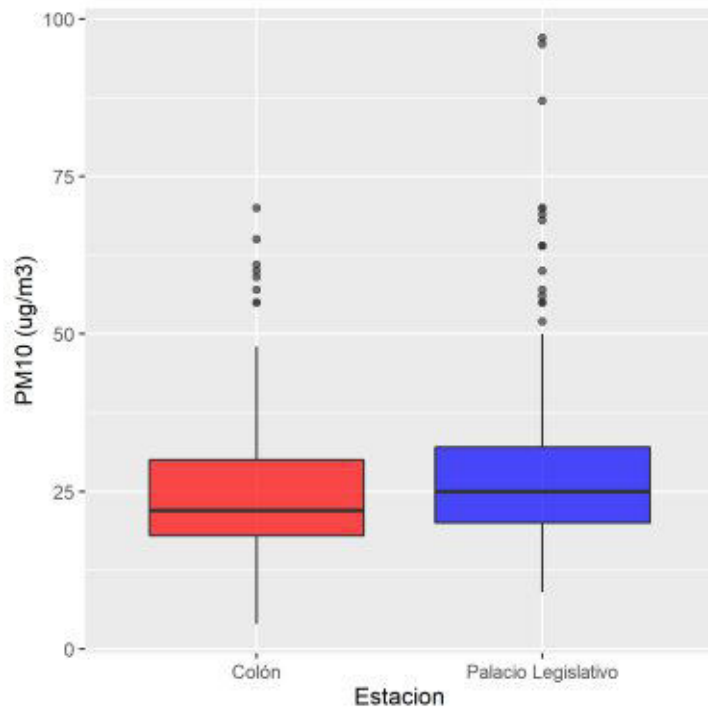
Ilustración 3.5 - Gráfico de cajas PM10 2020 por estación
