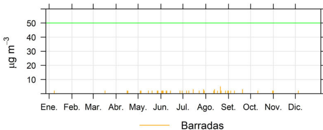
Ilustración 2.25 - Resultados SO 2 de la estación Barradas
