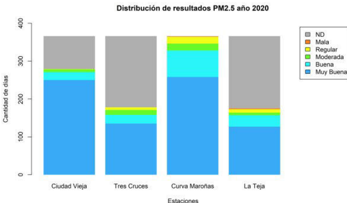
Ilustración 3.8 - Distribución por categorías PM2.5 2020 por estación
