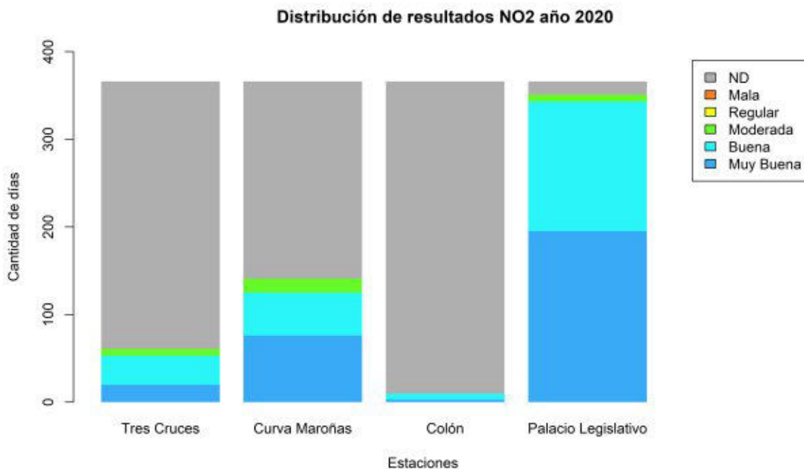
Ilustración 3.14 - Distribución por categorías NO2 2020 por estación
