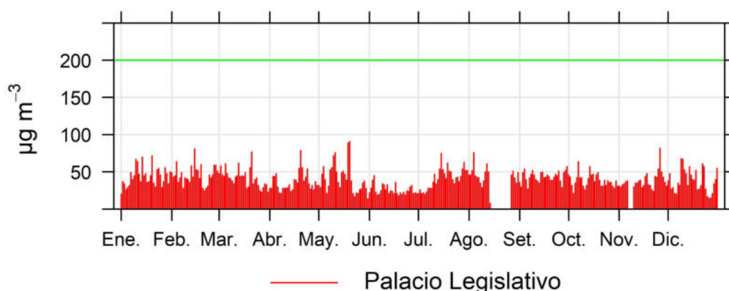
Ilustración 2.18 - Resultados NO2 de la estación Palacio Legislativo
