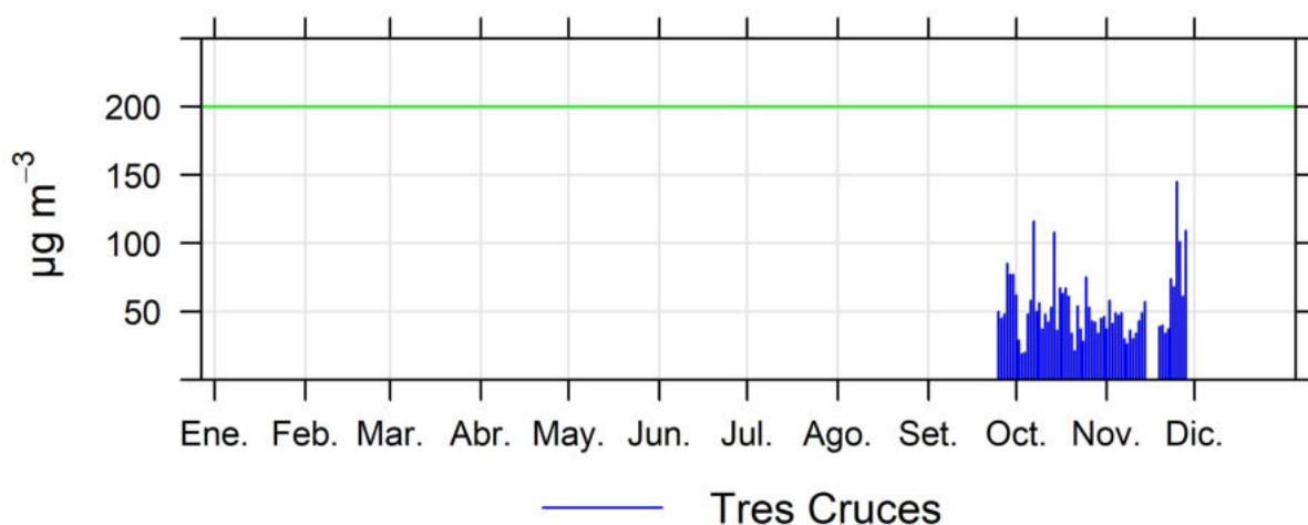
Ilustración 2.4 - Resultados NO 2 de la estación Tres Cruces
