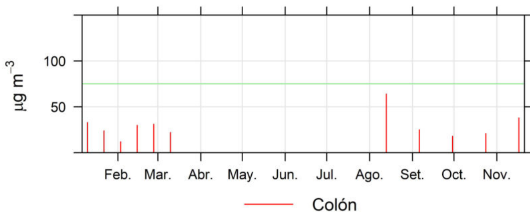
Ilustración 2.15-Resultados PM10 (manual) de la estación Colón
