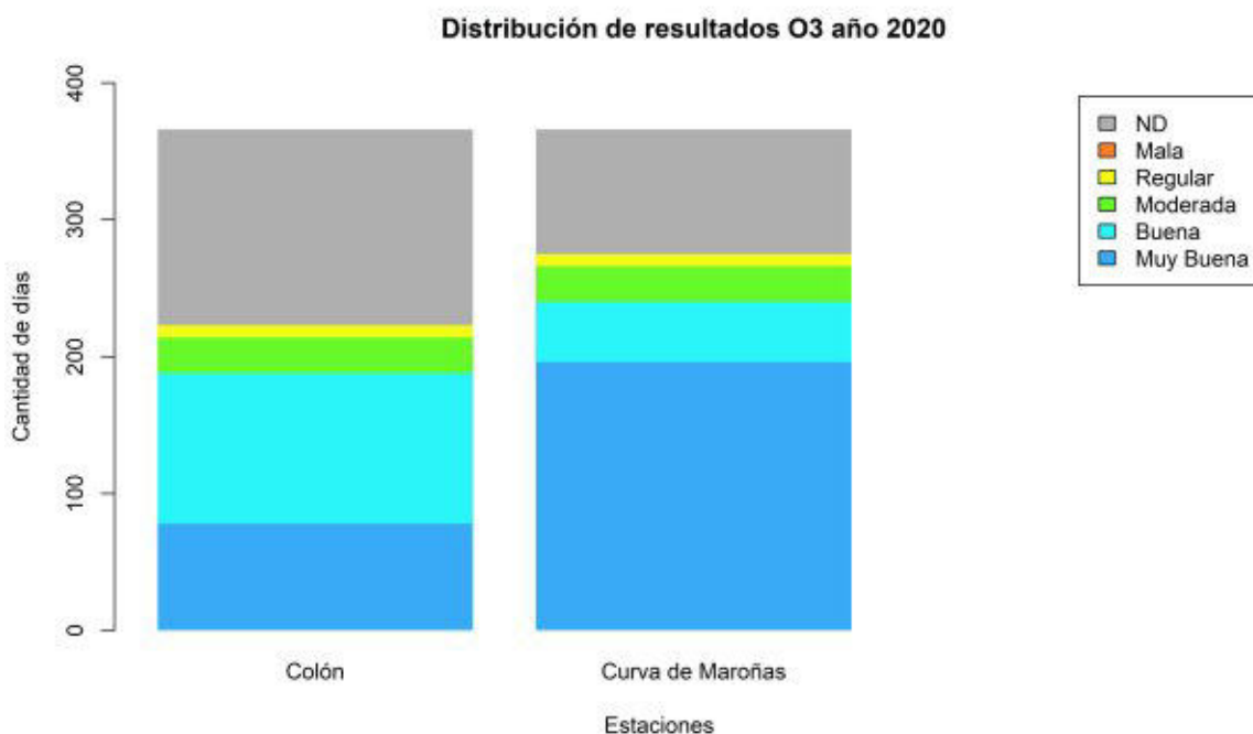
Ilustración 3.20 - Distribución por categorías O3 2020 por estación
