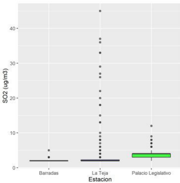
Ilustración 3.11 - Gráfico de cajas SO 2 2020 por estación
