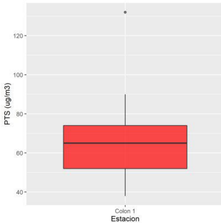
Ilustración 3.1 - Gráfico de cajas PTS 2020 por estación
