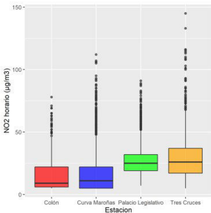
Ilustración 3.13 - Gráfico de cajas NO 2 2020 por estación
