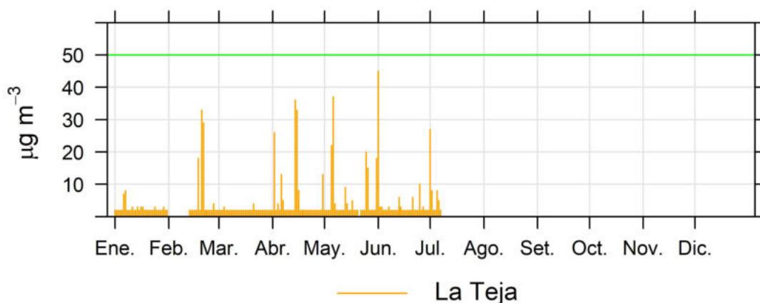
Ilustración 2.23- Resultados SO 2 de la estación La Teja
