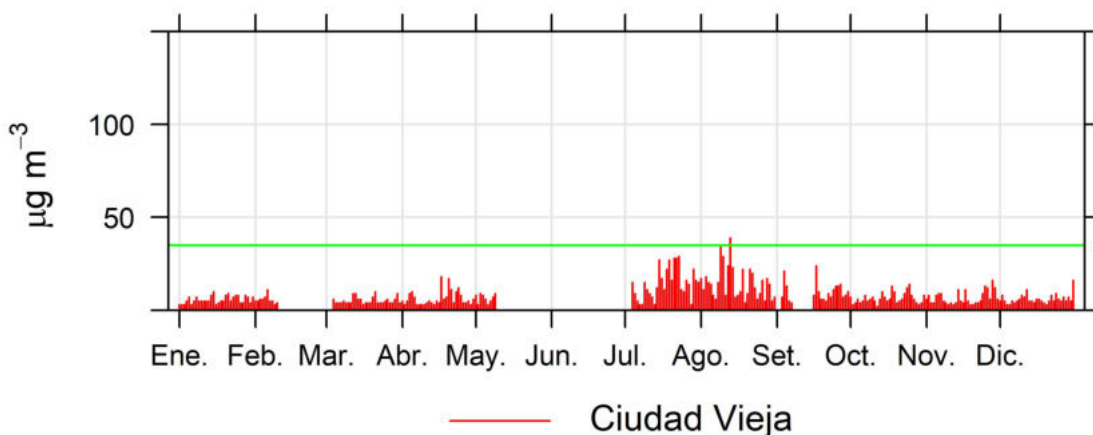
Ilustración 2.2 - Resultados de PM2.5 de la estación Ciudad Vieja
