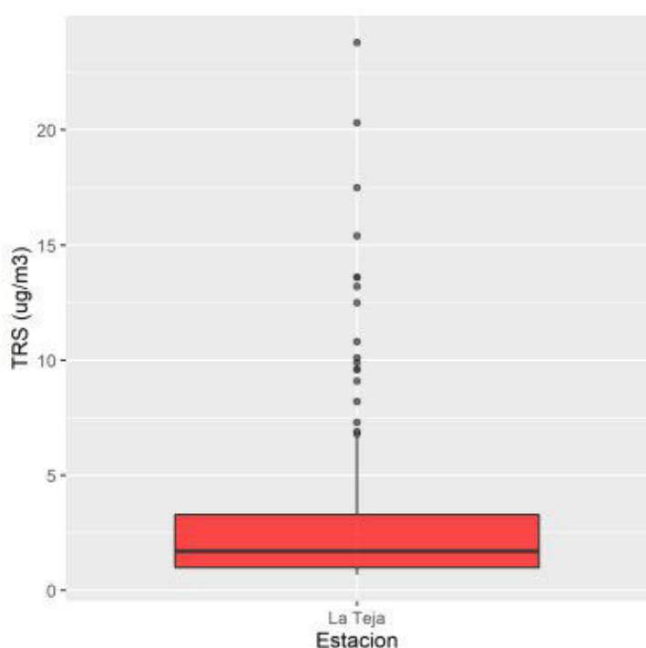
Ilustración 3.17 - Gráfico de cajas TRS 2020 por estación
