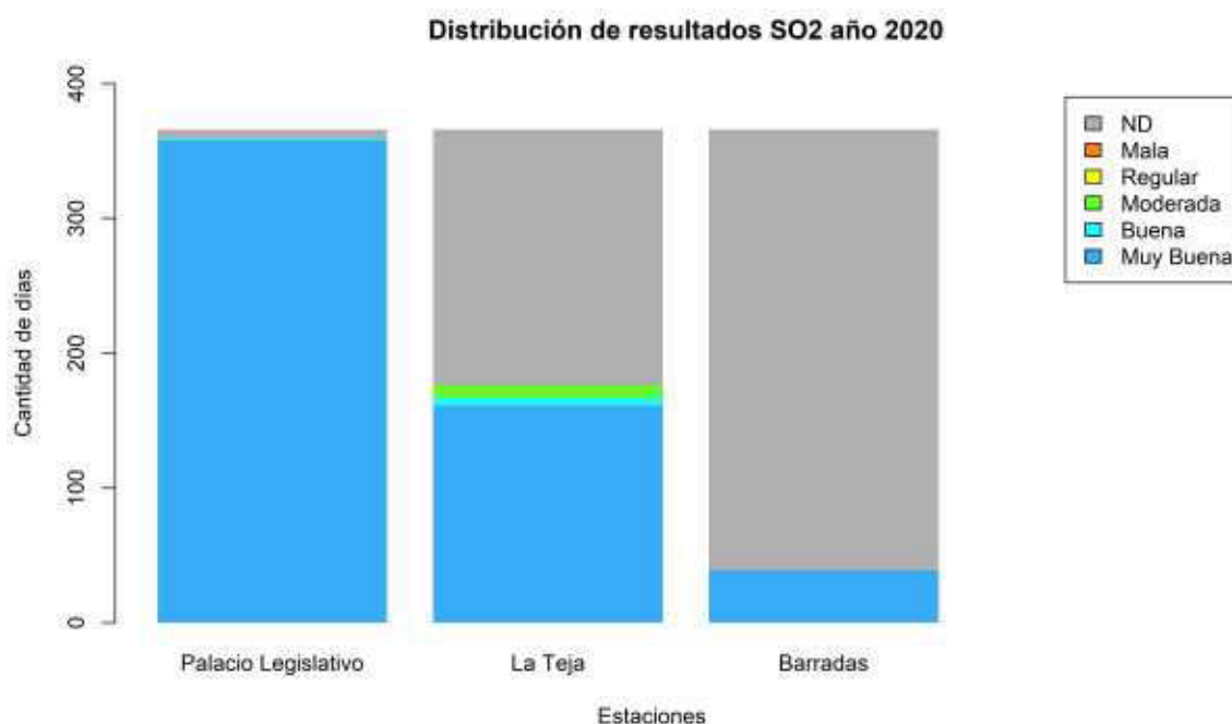
Ilustración 3.12 - Distribución por categorías SO2 2020 por estación
