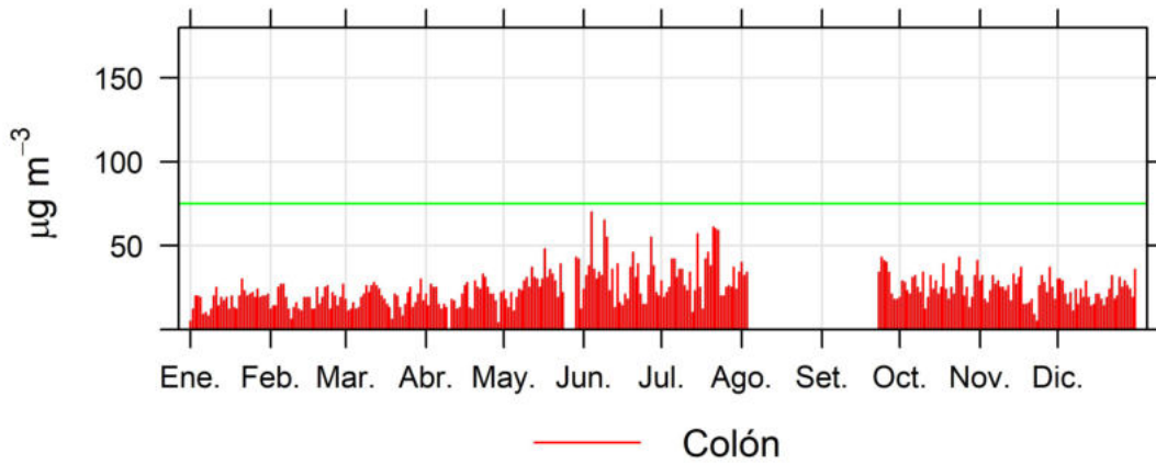
Ilustración 2.12- Resultados PM10 de la estación Colón
